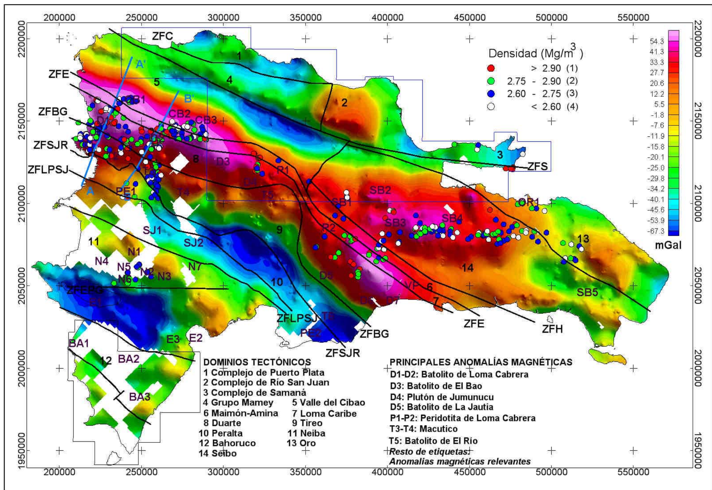
Figura 6. Anomalia de Bouguer de la República Dominicana. Se indica la posición de muestras sobre los dominios tectónicos y principales anomalías magnéticas. Coordenadas UTM en m, Huso 19 N. Distribución de densidades: (1) Eclogitas, gabros, anfibolitas, diabasas y rocas ultrabásicas; (2) Andesitas, basaltos y dioritas; (3) Dacitas, tobas básicas, tonalitas, esquistos y gneises; (4) Rocas ígneas ácidas (granitos, riolitas, tobas) y pizarras.
